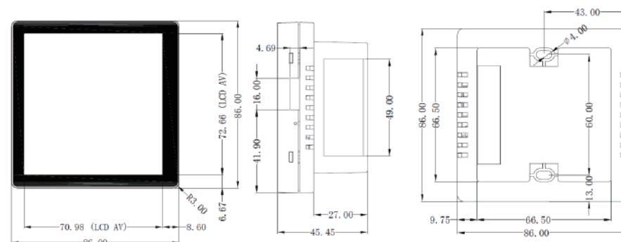
4、尺寸图示
